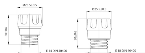
E 14 DIN 40400
