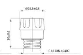
E 18 DIN 40400
