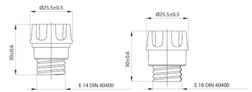
E 14 DIN 40400
