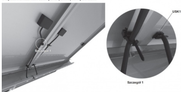
Przykład montażu kabli solarnych za pomocą uchwytów UKS1
