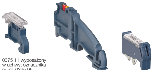
0375 12 z oznacznikiem CAB 3
