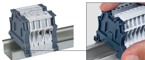
Oslona końcowa nr ref. 0375 10 – montaż bez użycia wkretaka
