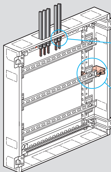
Demontowalna konstrukcja wsporcza
