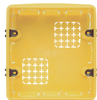
506E (108 x 118 x 51,5 mm) podtynk
