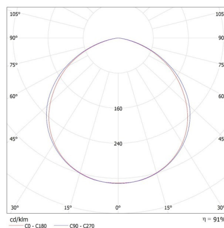
MILED o (kat 31394) GRUN NV LED-100-B / LDC (Polar)
