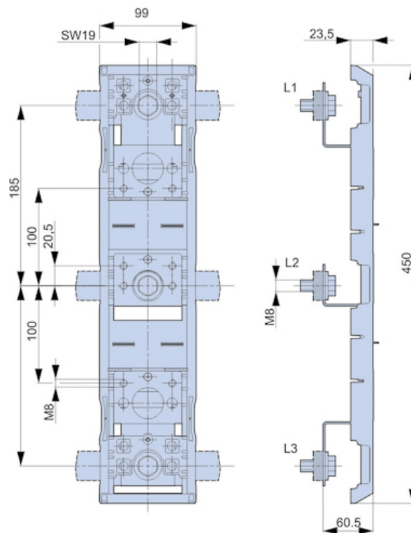
adapter DA 185-100/60
