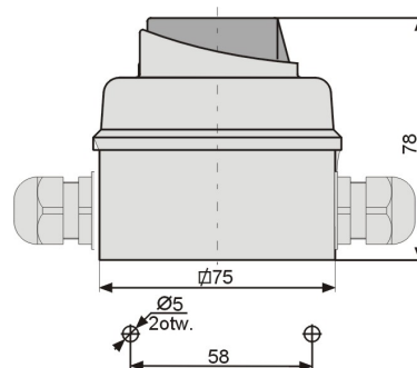
Rozłącznik 3 faz 0-I
