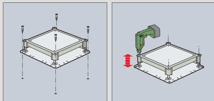
Mocowanie ramy
