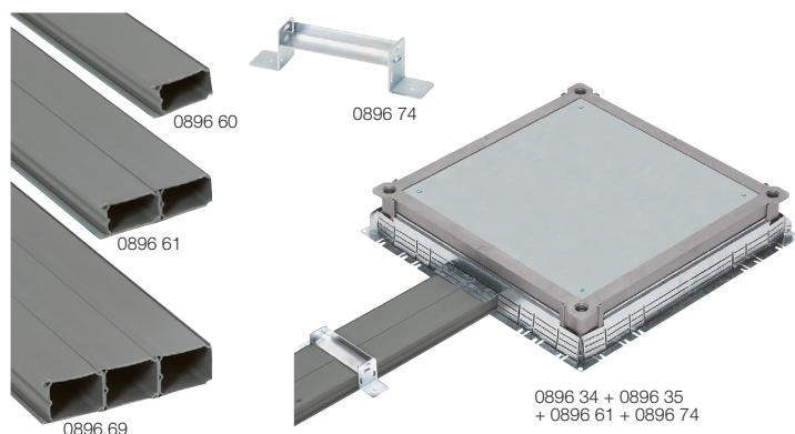
Mocowanie ramy
