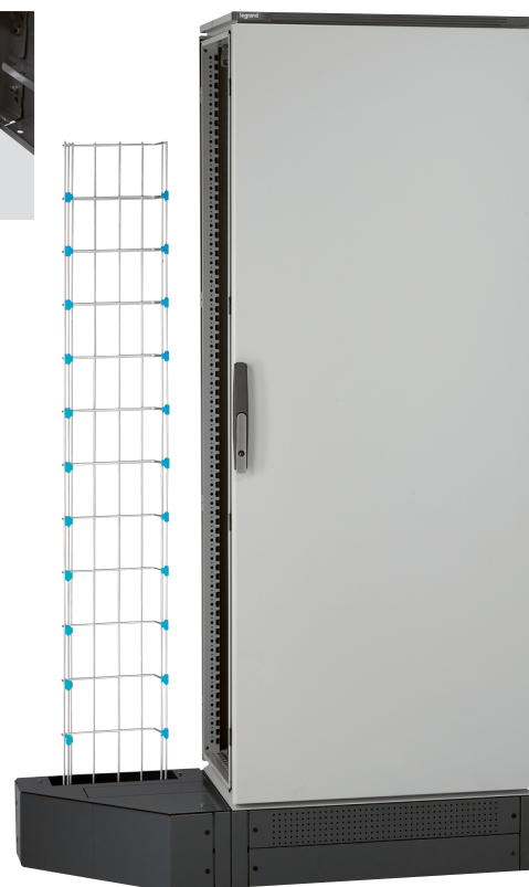
Przykład szafy zmontowanej z interfejsem 0477 05, korytkiem perforowanym do prowadzenia kabli i kompletnym cokolem z panelami pełnymi
